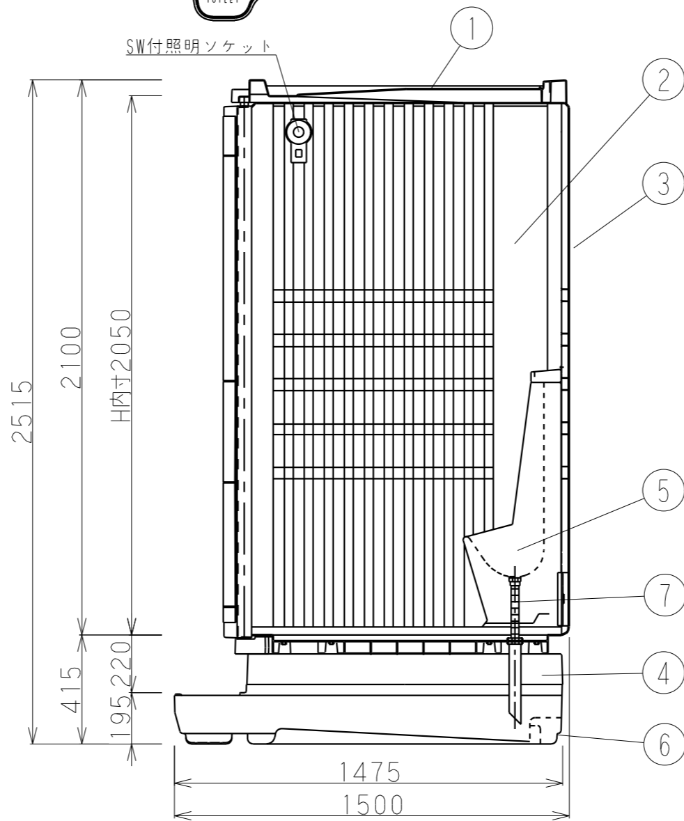
側面図
