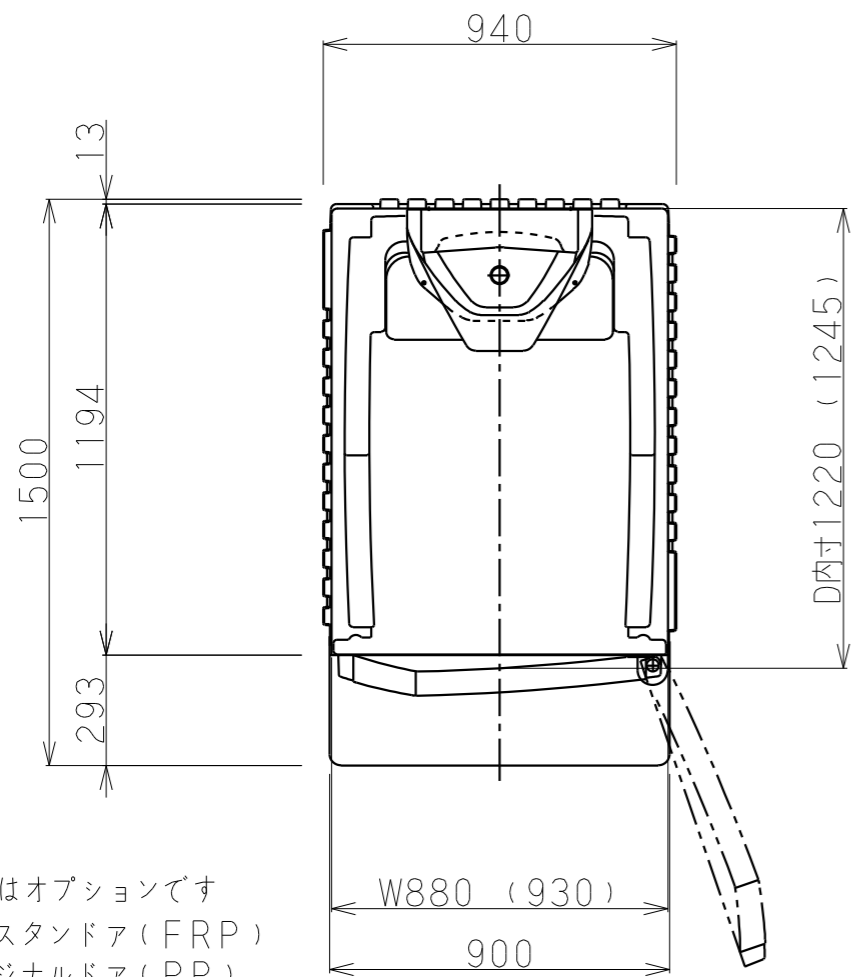
平面図
