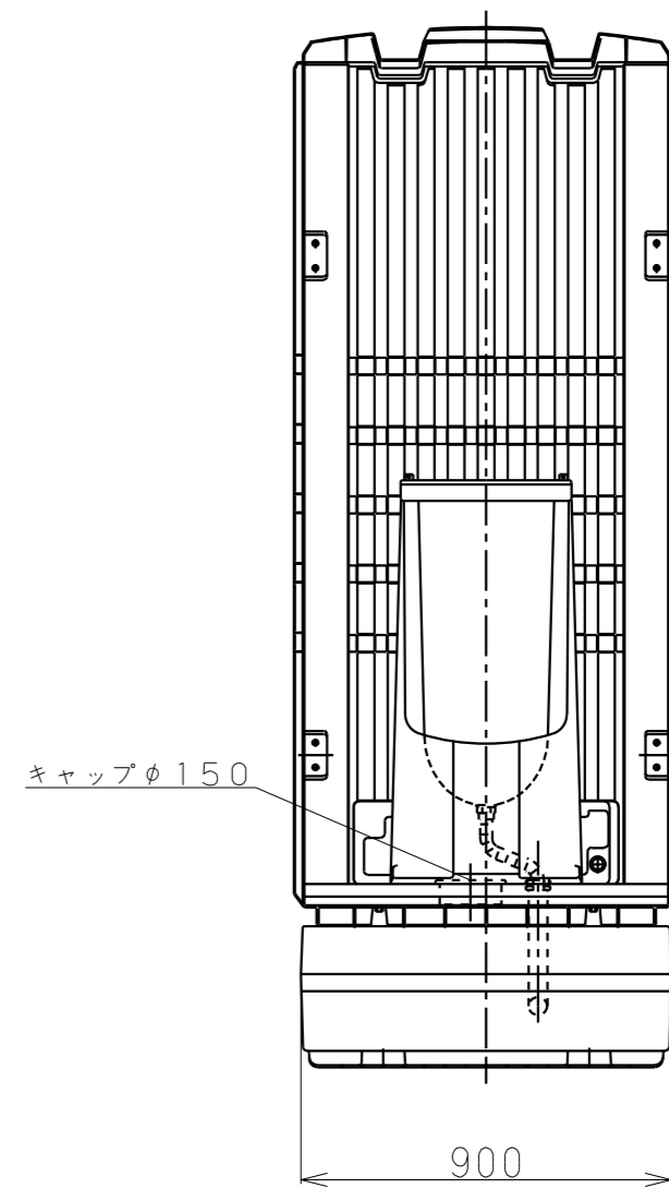
正面図
