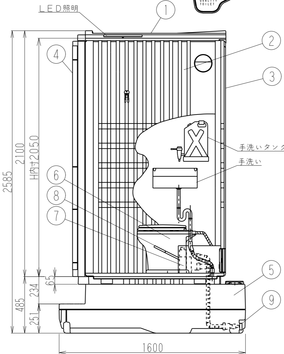
側面図
