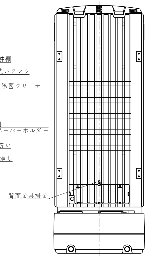
背面図
