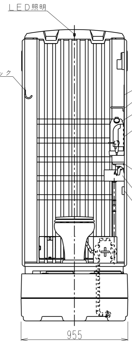
正面図
