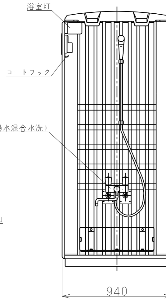
正面図
