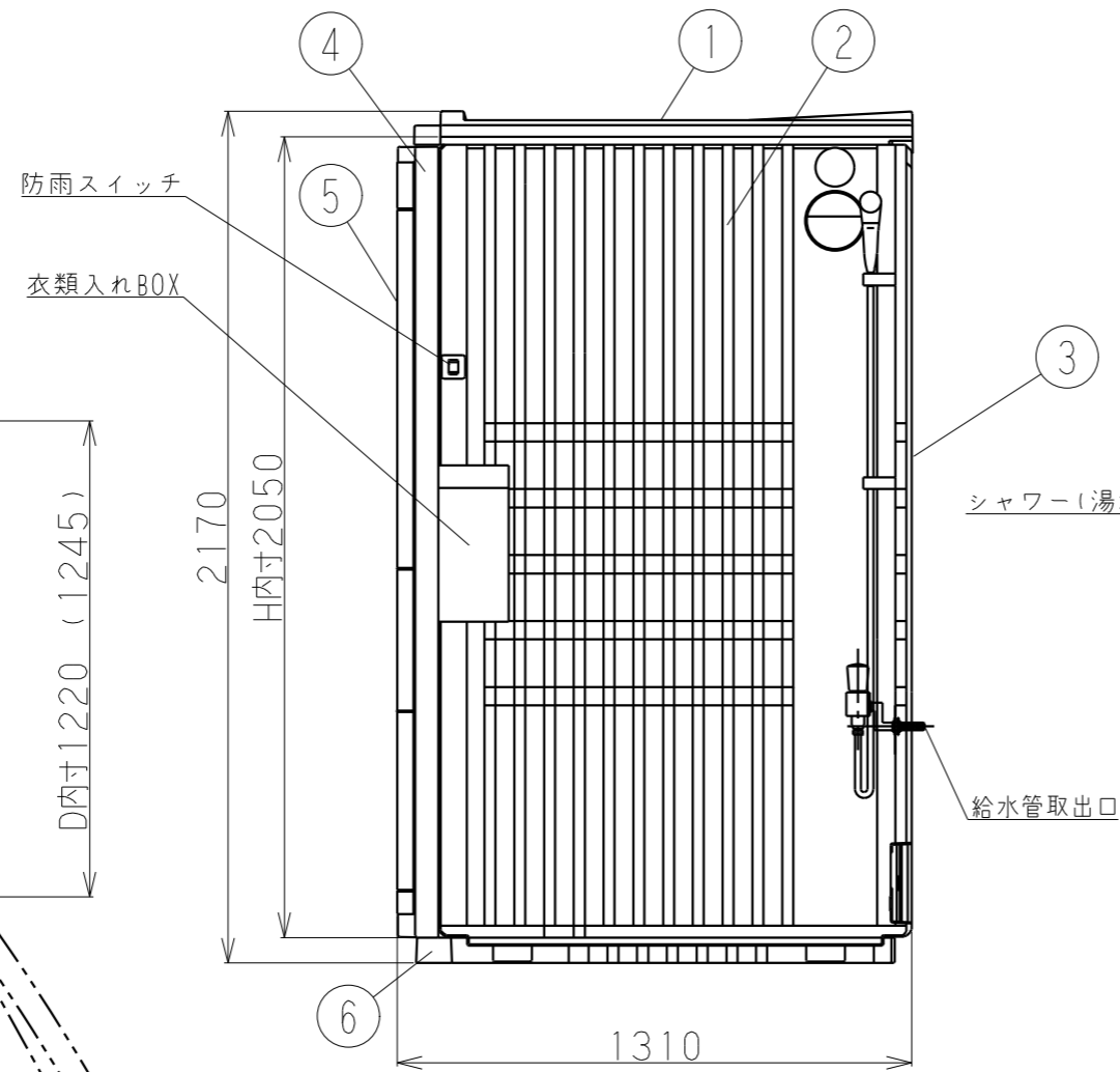
側面図
